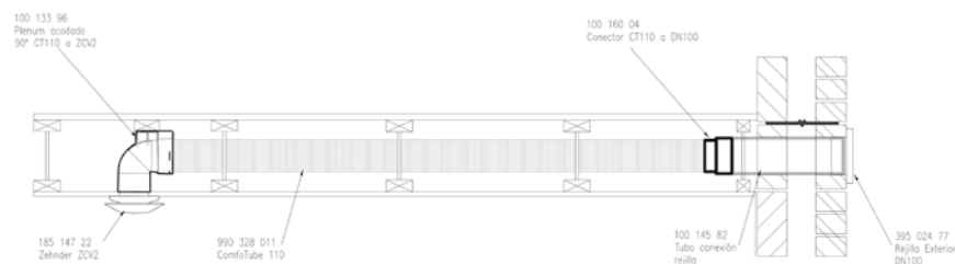
Ejemplo de conexionado de accesorios
